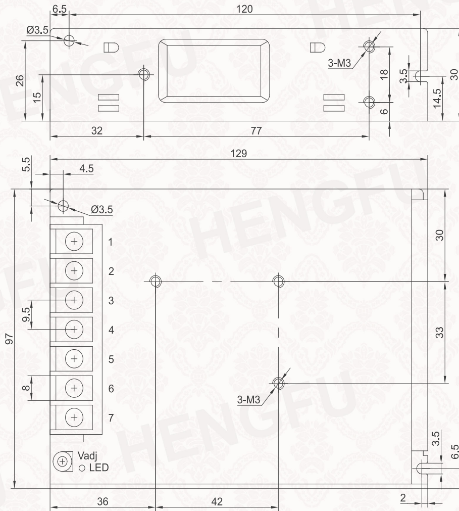
机壳 Frame
